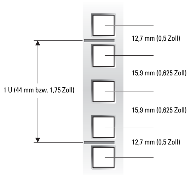
Abbildung 3-3. Eine Rack-Einheit
